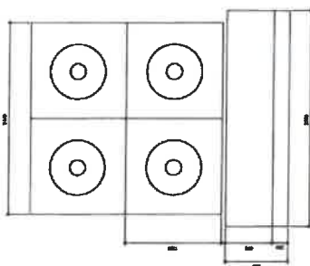
ELEVATION B - B
